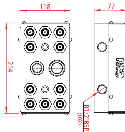
• Acoplador Troca Rápida 5x5 E2-5 Bloco Lado Molde
